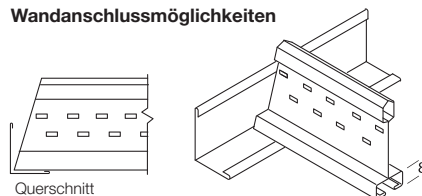
Silhouette Schiene auf L-Wandwinkel
