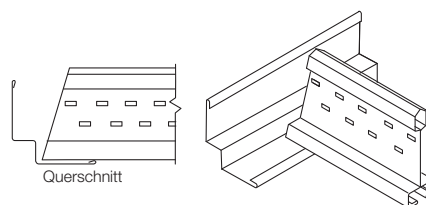
Silhouette Schiene auf Stufenwandwinkel BPT 1508 HB (Seite 46) aufgelegt.
