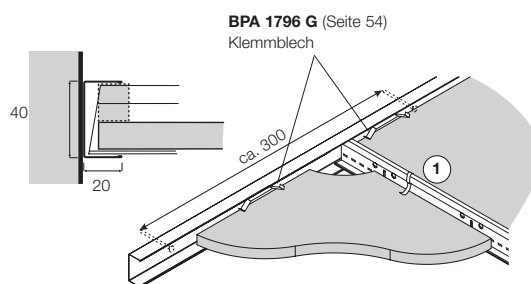
Wandanschluss mit U-Wandwinkel BPT 2040 HA ① BPA 7890 G Universal Plattenfeder
