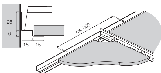
Wandanschluss mit Schattennut, Tegular BPT 1506 H
