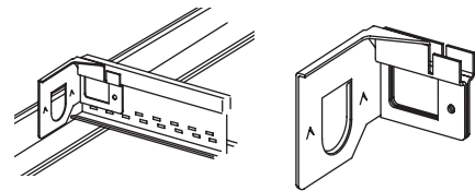
BERC (attache de retenue de bout de longeron) Joint l'âme du longeron principal ou du té croisé à la moulure murale sans rivets pop apparents
