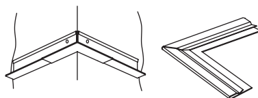
7865 (couvre-coin extérieur) Pour moulure à angle de 9/16 po nom.; s'enclenche sur la moulure pour garnir les coins extérieurs; pattes de 2 po
