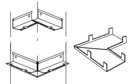
7869 (couvre-coin intérieur/extérieur) Pour moulure à angle de 7/8 po nom.; pattes de 1 3/4 po
