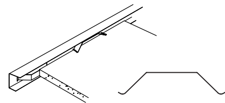
7870 (attache à ressort) Attaches de bordure à poser entre les carreaux de plafond et les fixations de périmètre
