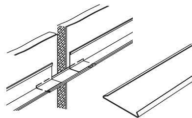
ES4 (manchon d'expansion de 4 po) Manchon d'expansion pour longerons principaux, tés croisés et moulures murales à angle de 15/16 po; couvre les joints d'expansion, les trous de vis sur la face du treillis et les rainures des longerons principaux
