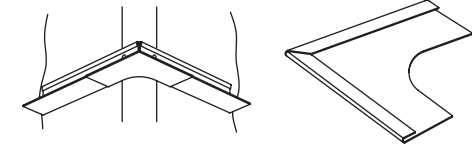
7866 (couvre-coin arrondi) Pour moulure de 15/16 po nom.; s'enclenche sur la moulure pour garnir les coins extérieurs; convient aux blocs de 1 po de rayon; pattes de 2 po
