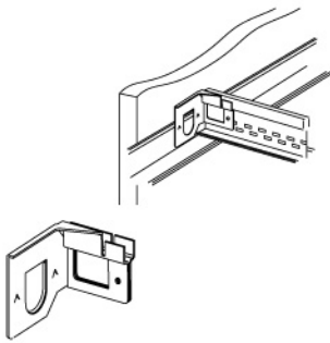
BERC - 龙骨头部固定夹 将主龙骨或副龙骨与边龙骨连接在一起，并且使整个龙骨的框架结构没有可见的铆钉。
