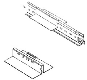
EHDC50 - 外部压紧夹，用于1/2英寸平板式天花板和干墙 EHDC58 - 外部压紧夹，用于5/8英寸平板式天花板和干墙 EHDC75 - 外部压紧夹，用于3/4英寸平板式天花板和干墙 在龙骨的头部下面的锁住，以防天花板上移，符合UL15和90等级。
