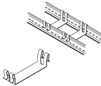
ABSC - 空间杆间隔夹 使主龙骨保持平行的固定夹，以使通风口与龙骨更均匀地分布。可提供的尺寸是1-7/8英寸到6英寸，每隔1/8英寸增加一个规格。
