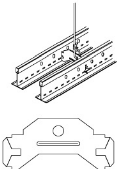
MBSC2 - 主龙骨间隔夹(2英寸长) 用来间隔两根平行的主龙骨以便于通风。常规尺寸为4英寸中心距。
