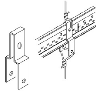
DLCC - 天花板直接承载夹子 适用于吊装现有的低于24mm宽度的龙骨悬吊系统，将负载直接地传到悬吊钢丝上，这有利于保持现有的天花系统耐火时间，适用于悬吊重型附件(参考当地的标准而选择)。
