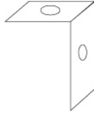
BPGM2626 - 直角钢丝吊钩 一边固定膨胀螺栓上，另一边用于悬吊钢丝。
