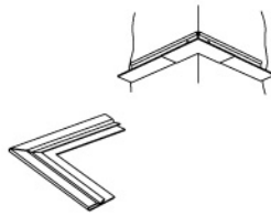
7865 - 外角护套 适用于常规的15毫米宽边龙骨，以使边龙骨两端直角连接处外部更整齐。
