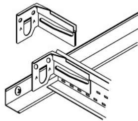
BERC2 - 龙骨头部固定夹
