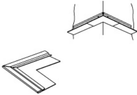
7863 - 外角护套 适用于常规的22毫米宽边龙骨，以使边龙骨两端直角连接处外部更整齐。
