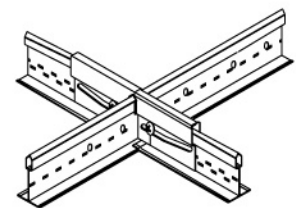
SJCG - 副龙骨/主龙骨连接件
